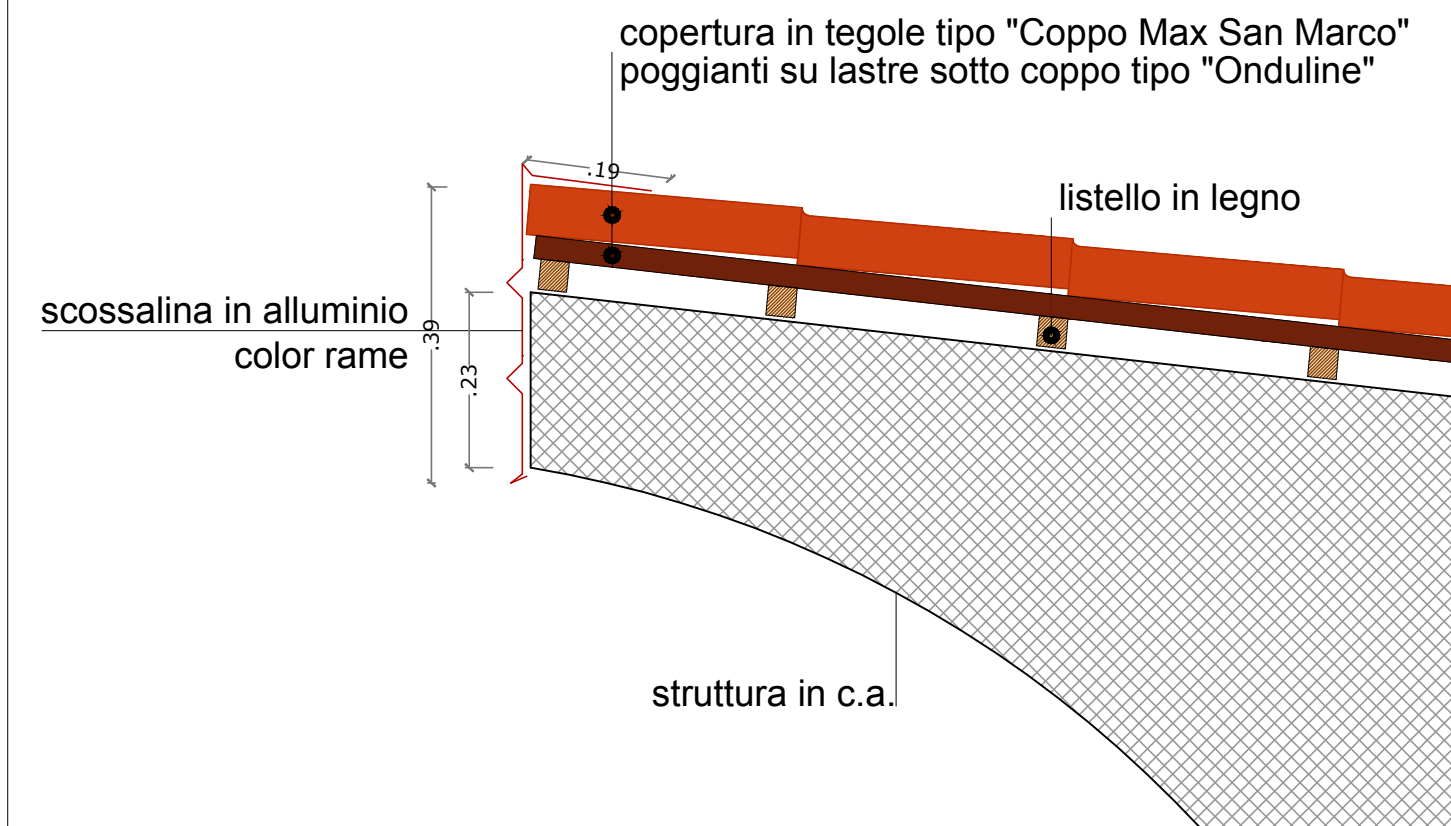
PARTICOLARE 3
