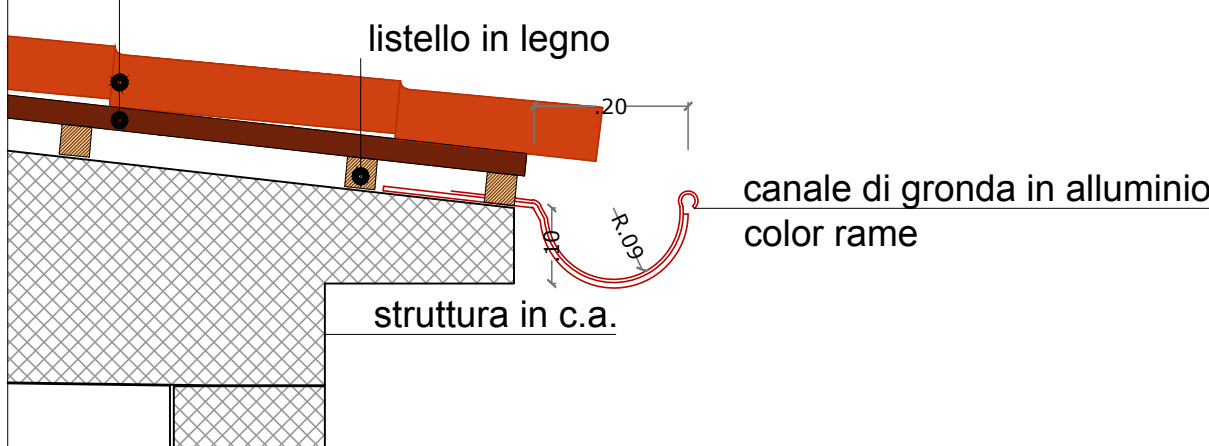
PARTICOLARE 2
