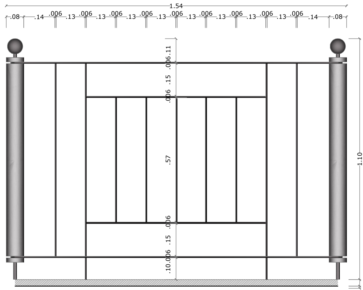
prospetto ringhiera
