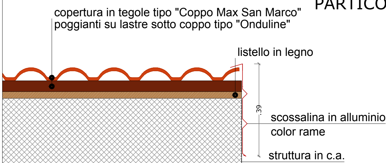
PARTICOLARE 3
