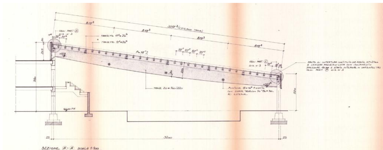
Fig.1,7: sezione copertura vasche
