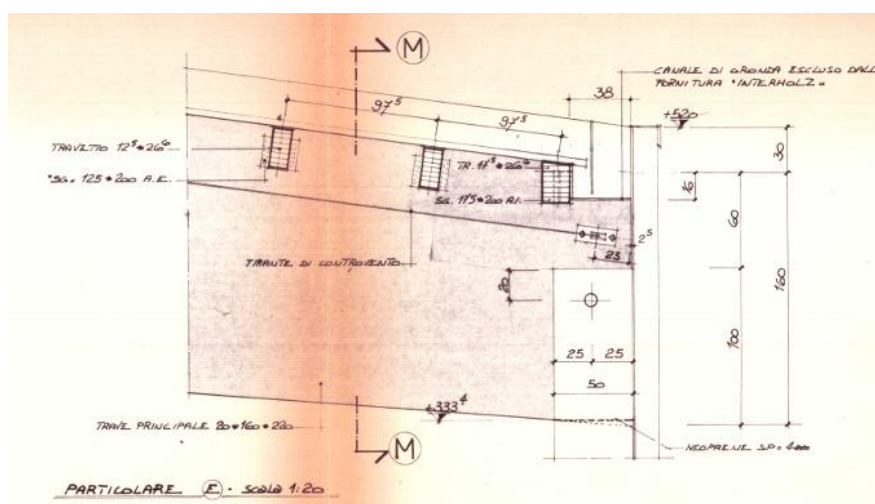
Fig.1,8: dettaglio appoggio travi su colonne
