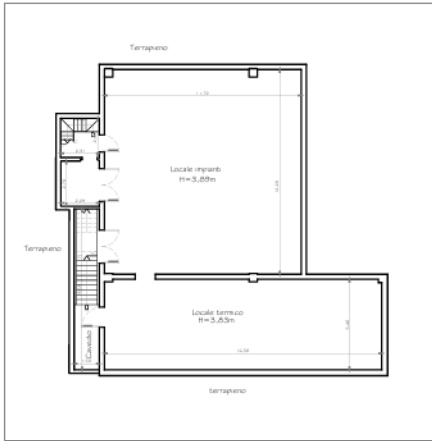
Fig.1,5: pianta piano interrato
