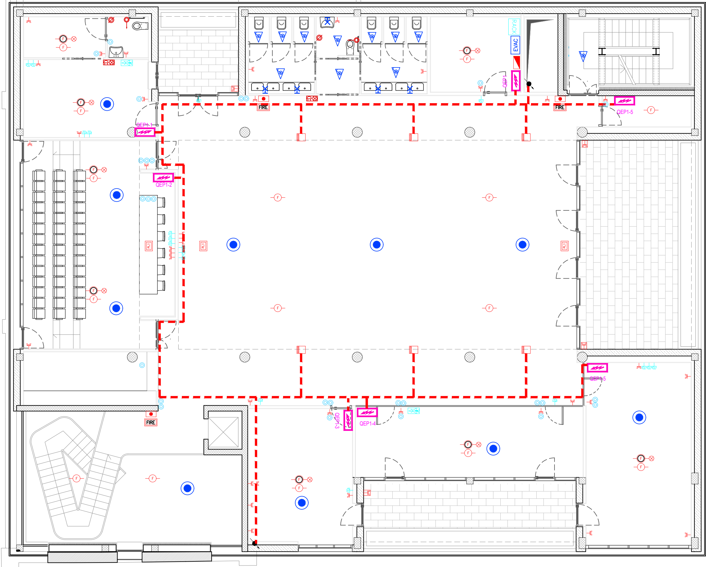
PIANO PRIMO SCALA 1:100
