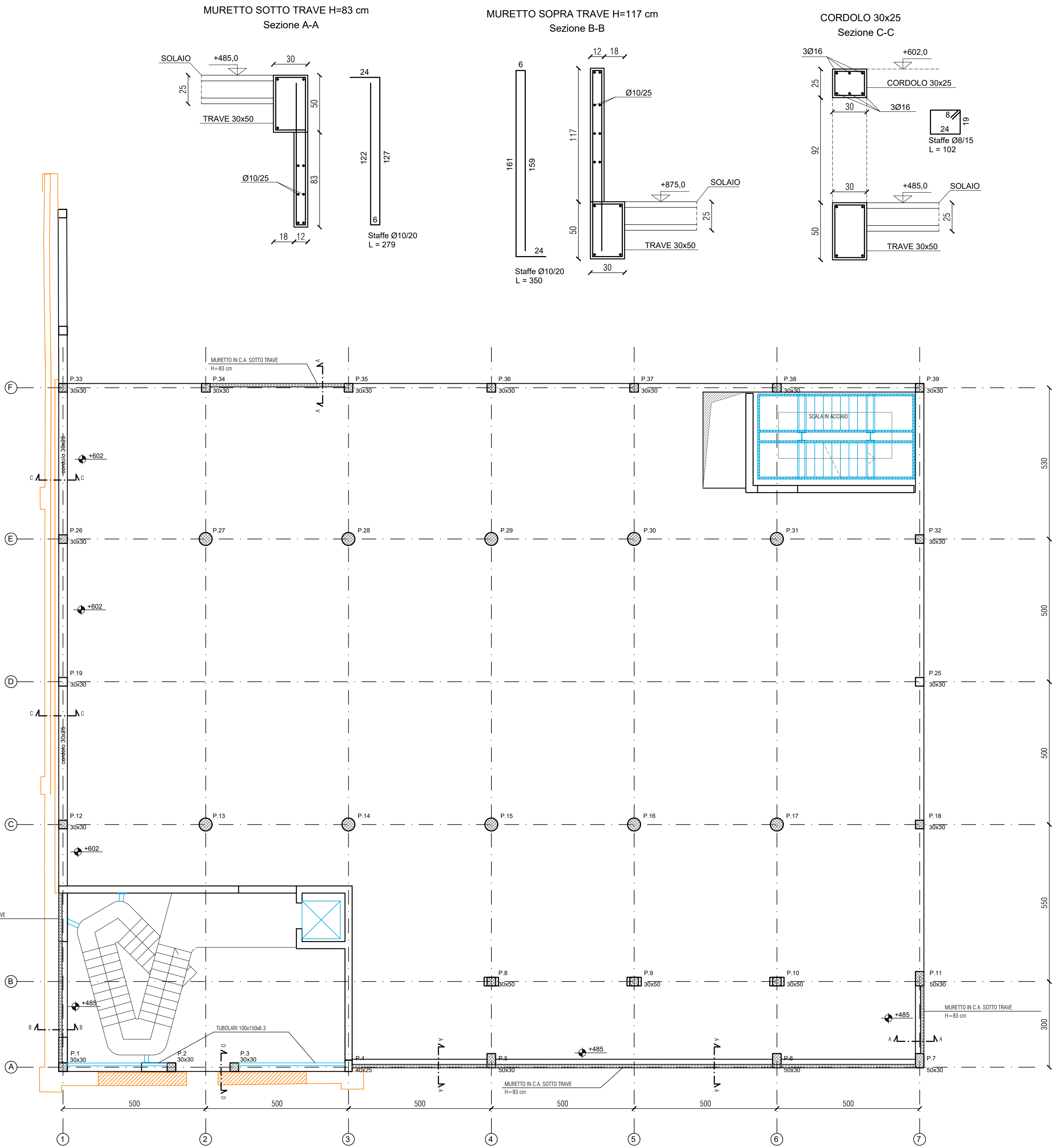
Pianta Muretti e cordoli Quota +4.85/+5.90
