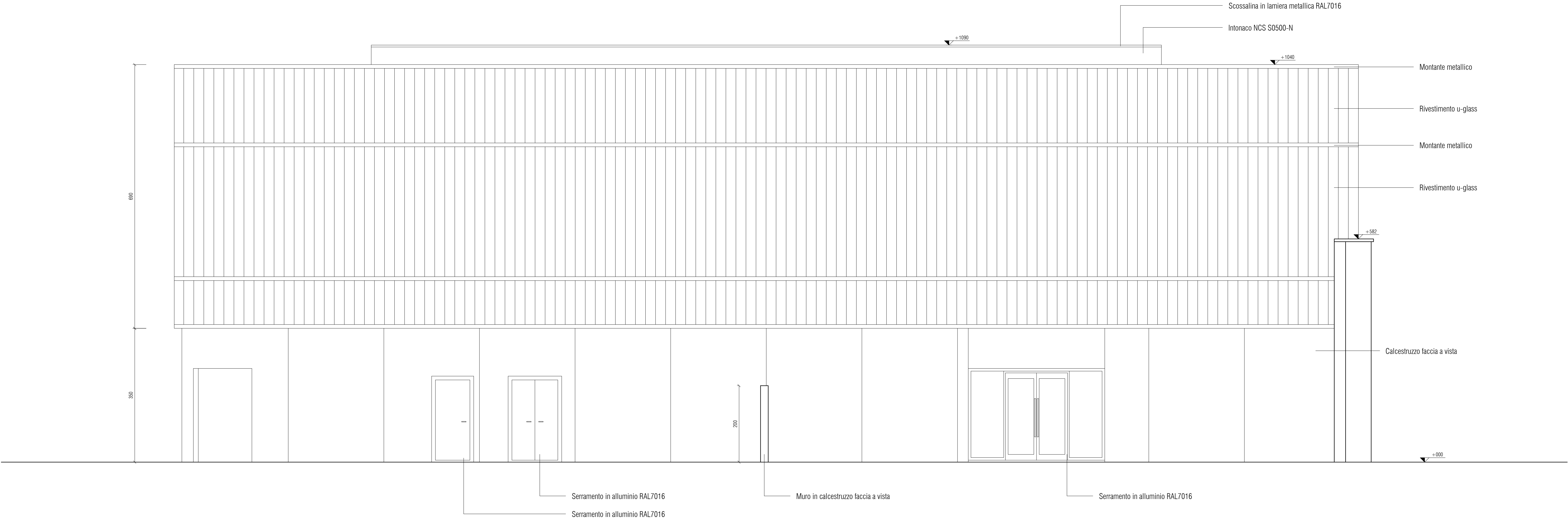
PROSPETTO NORDOVEST
