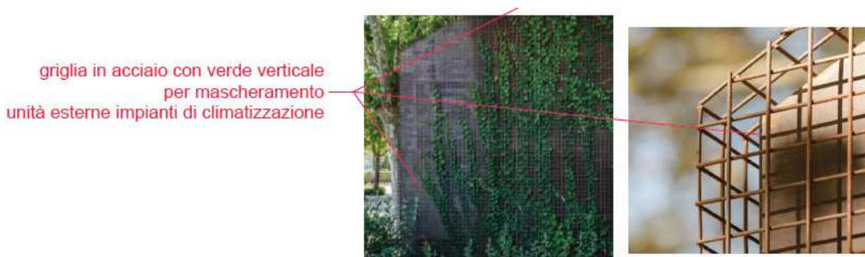
Particolare verde verticale su supporto in rete metallica
